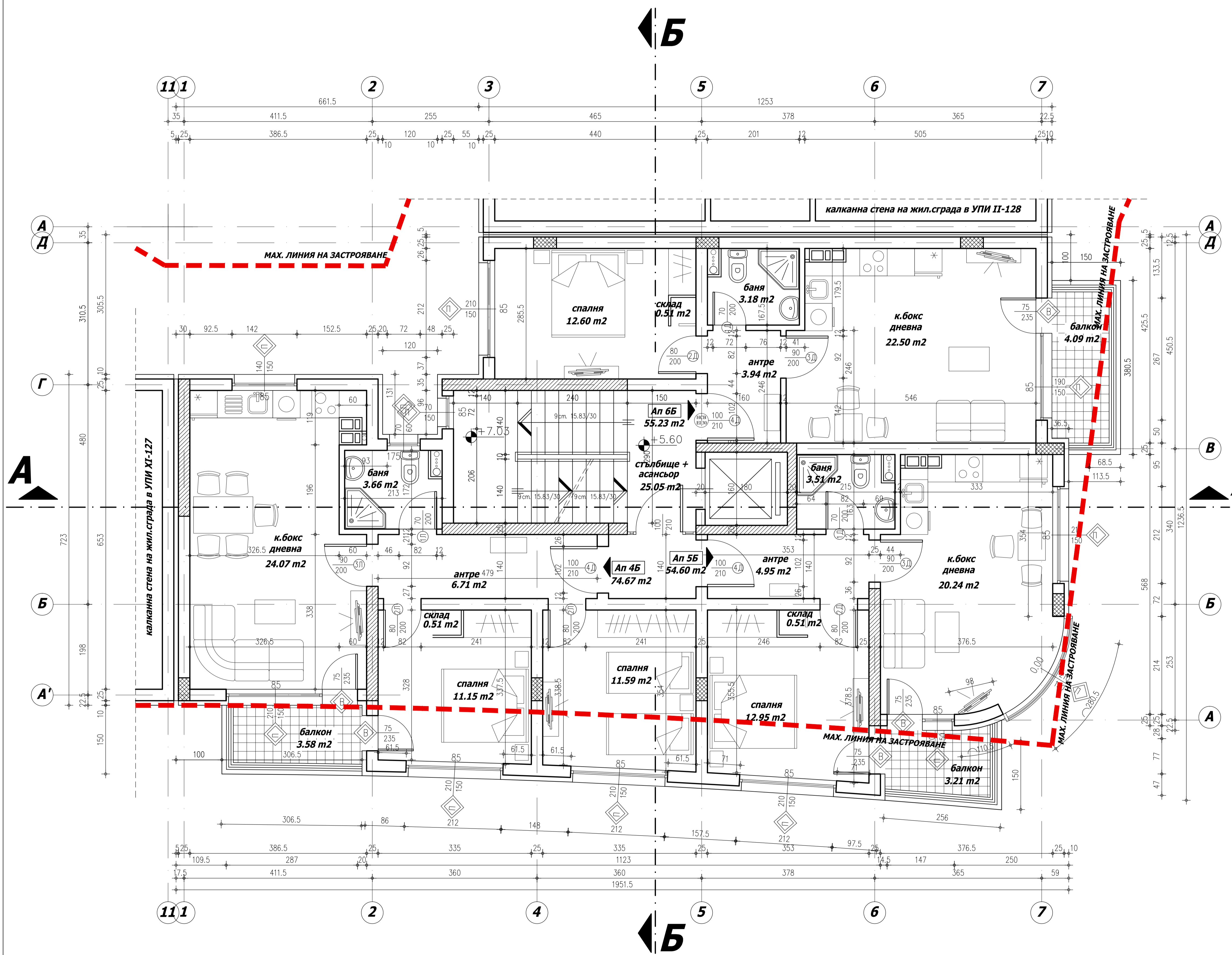
РАЗПРЕДЕЛЕНИЕ II ЕТАЖ М 1:50
