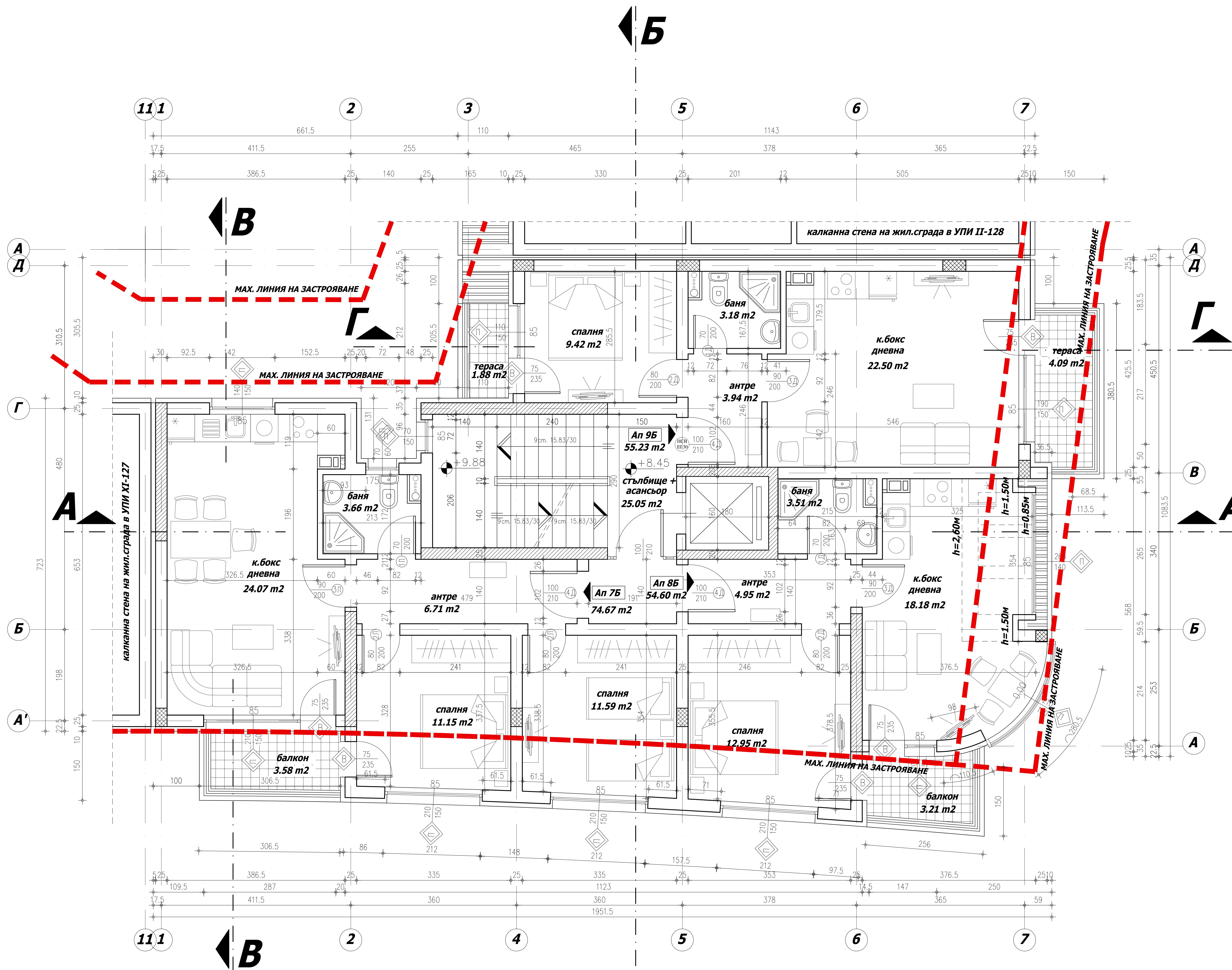
РАЗПРЕДЕЛЕНИЕ III ЕТАЖ М 1:50
