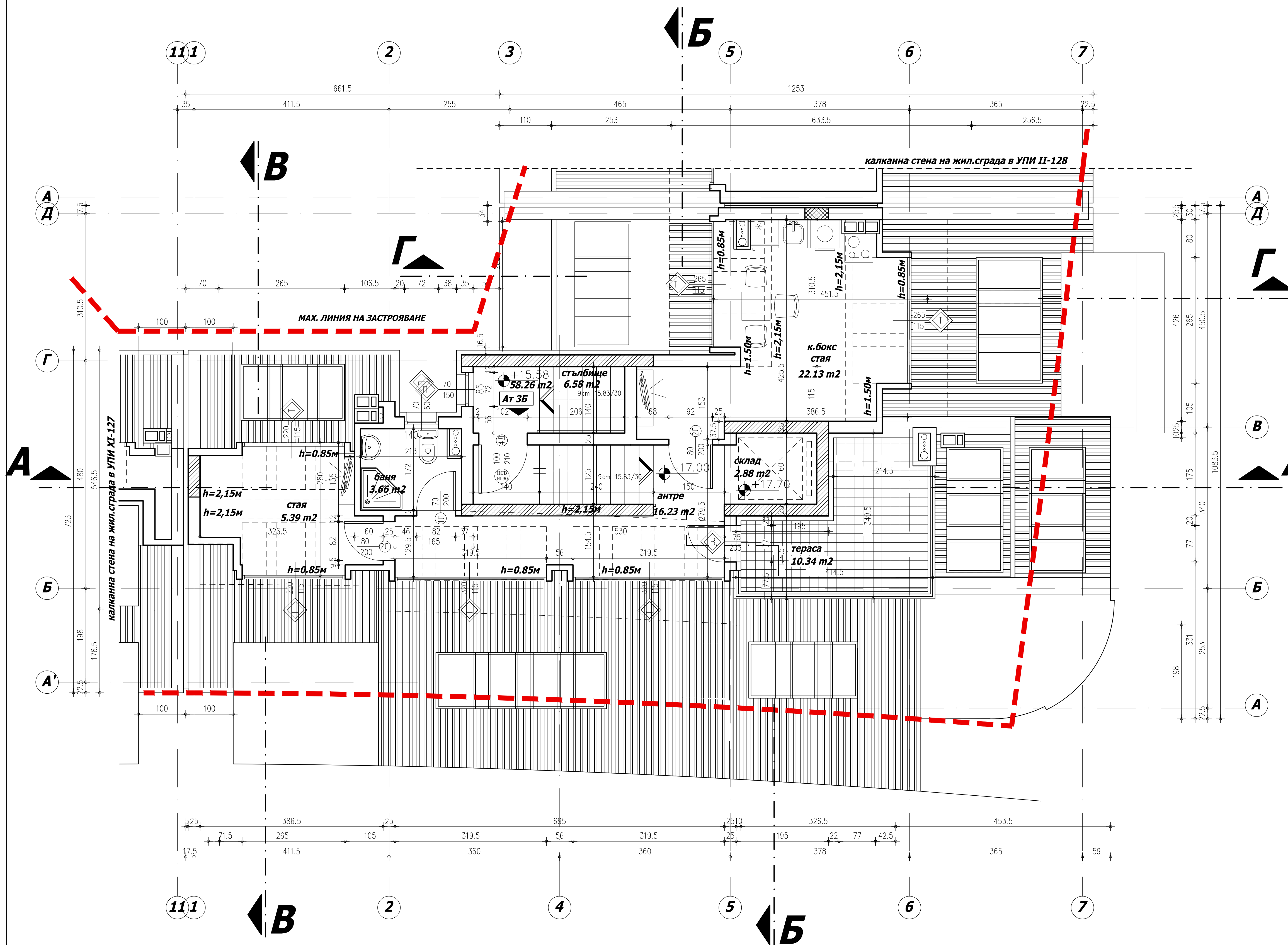
РАЗПРЕДЕЛЕНИЕ II ПОДПОКРИВЕН ЕТАЖ М 1:50
