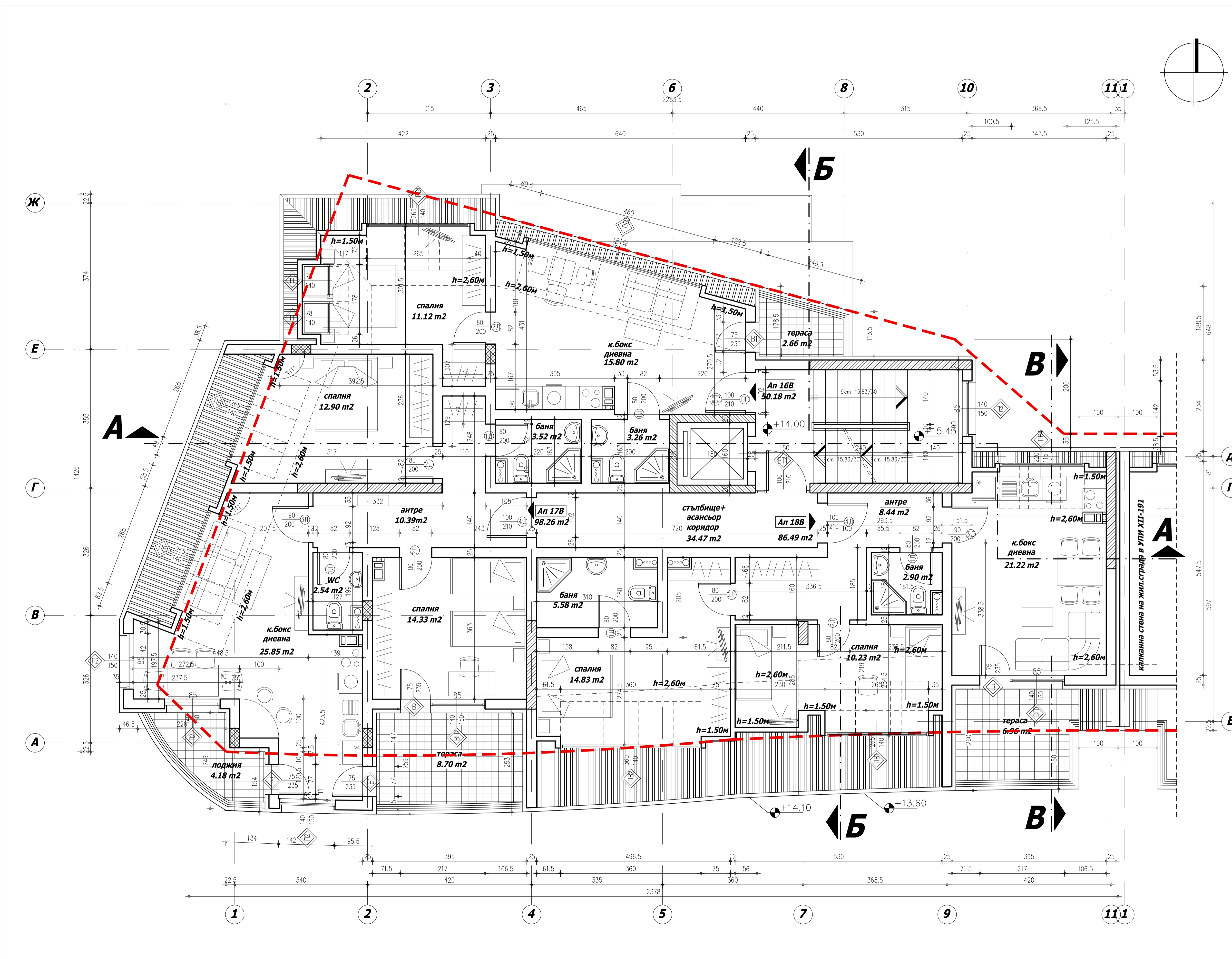
РАЗПРЕДЕЛЕНИЕ I ПОДПОКРИВЕН ЕТАЖ М 1:50
